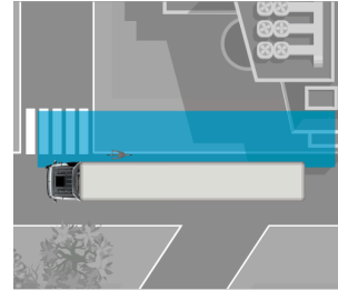
Actros mit Abbiegeassistent S1R (2 Nahbereichssensoren erfassen einen Bereich von 3,75 m Breite und 18,75 m Länge)
