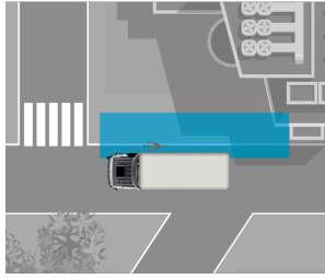
Atego mit Abbiege-Assistenzsystem, basic (1 Nahbereichssensor erfasst einen Bereich von 3 m Breite und 12 m Länge)
